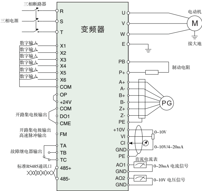
图3-4 基本配线图
