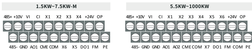
图3-6 控制板端子排列顺序图
