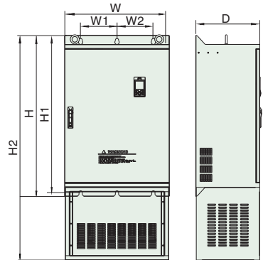
图2-10 加底座
