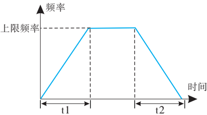
6-03 直线加减速
