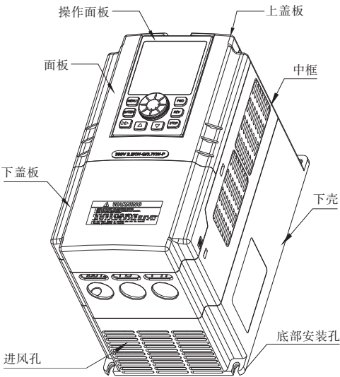
图2-3 产品结构外形图
