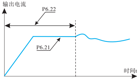
图6-28 PID初值功能示意图
