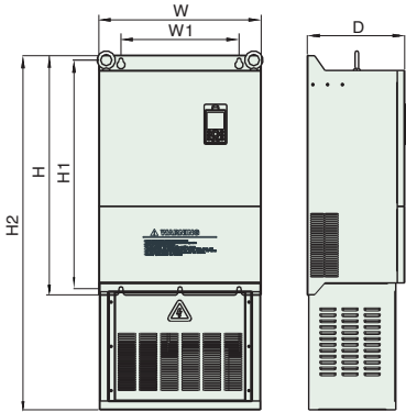
图2-6 加底座
