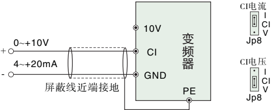
图3-8 CI端子配线图
