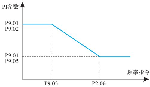
图6-32 PI参数示意图
