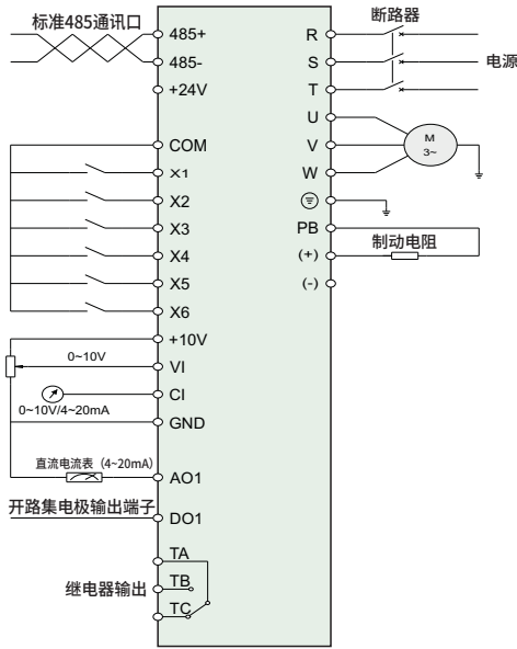
图3-4 基本配线图
