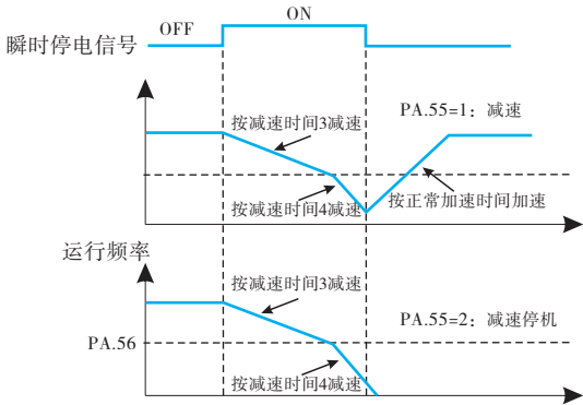
图6-34 FDT功能的电平示意图
