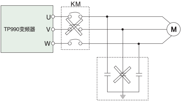
图1-1 变频器输出端禁止使用电容器
