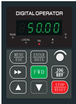
图B 停机状态，显示停机状态参数
