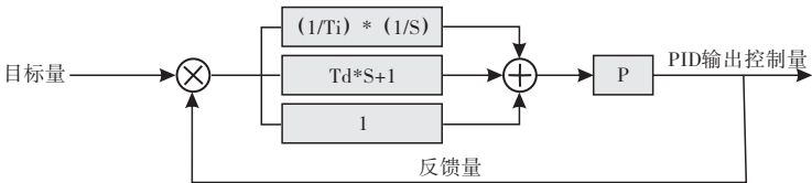
图6-26 过程PID原理框图
