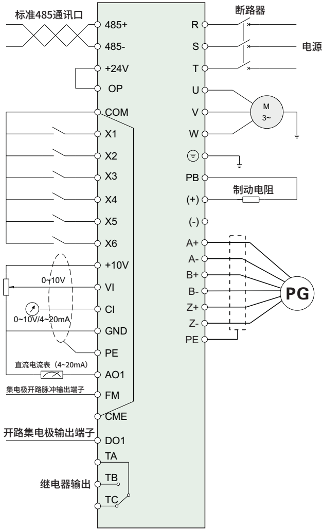
图3-5 基本配线图
