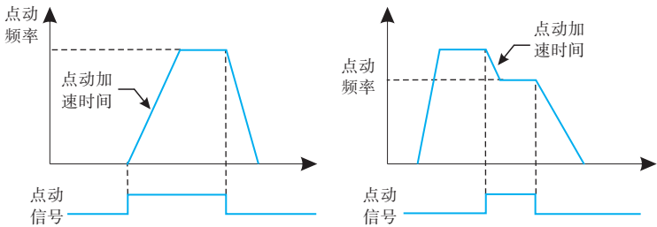
图6-05 点动运行
