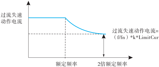
图6-38 倍速过流失速动作示意图
