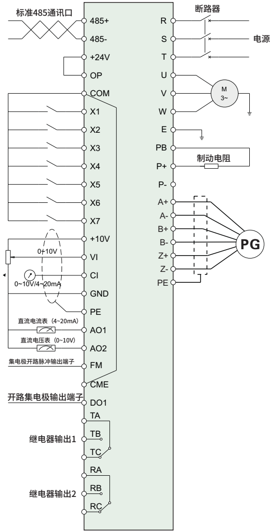
图3-6 基本配线图 (TP990-4T0300G, TP990-4T0370G)
