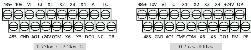
图3-8 控制板端子排列顺序图
