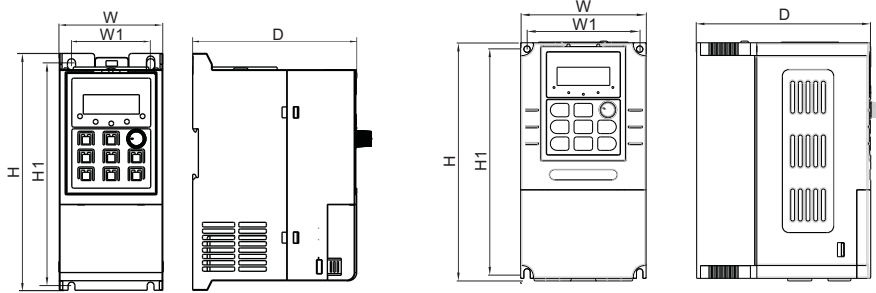
单相0.75G~3.7G / 三相0.75G~2.2G外观尺寸图
